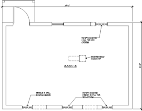
1 A1.0 EXISTING PLAN Scale: 3/8" = 1'-0"
