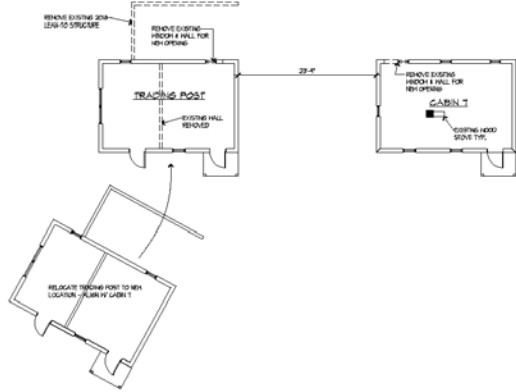
1 A1.0 EXISTING PLAN Scale: 3/8" = 1'-0"
